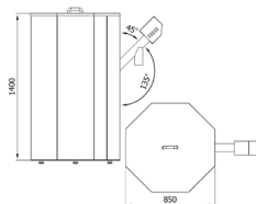
ZÁSOBNÍK 500 L.
