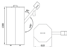
ZÁSOBNÍK 340 L.
