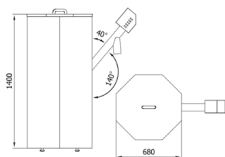
ZÁSOBNÍK 500 L.
