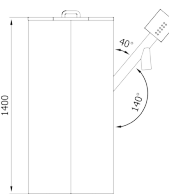
ZÁSOBNÍK 340 l.
