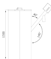
ZÁSOBNÍK 240 l.
