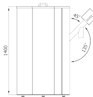
ZÁSOBNÍK 500 l.
